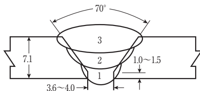
パイプの開先形状 (6 寸 × Sch 40)
